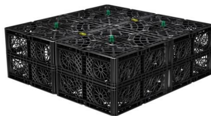
Obrázek 11: Vertikální spoj - středící kolíky a horizontální spoj - konektory EcoBloc
