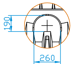
Detail nátku (1:20)
