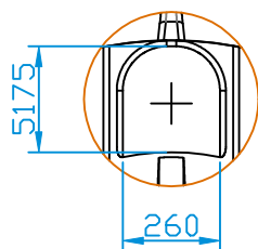
Detail nátku (1:20)
