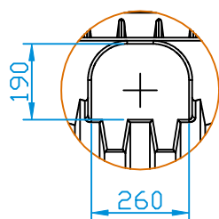
Detail nátku (1:20)
